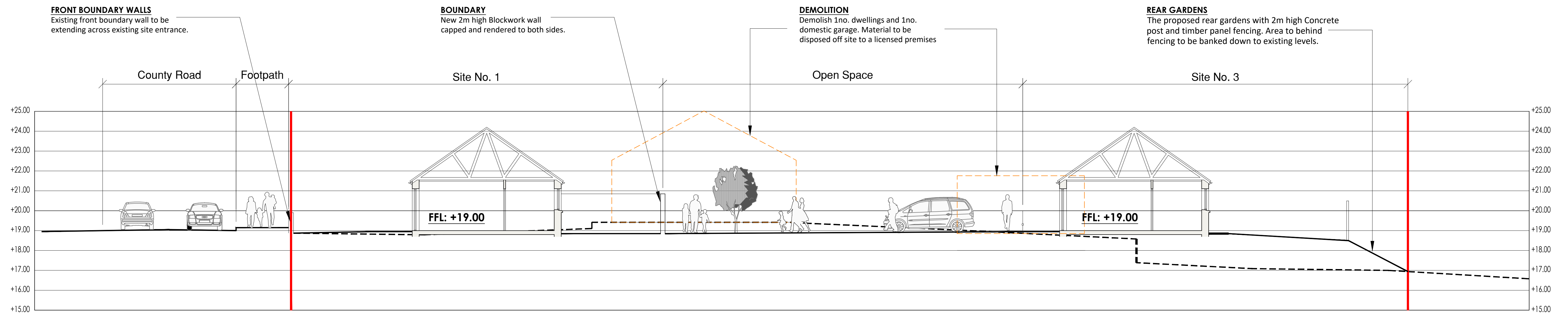
Site Section A-A Scale 1:100
